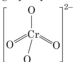
Chromate ion
