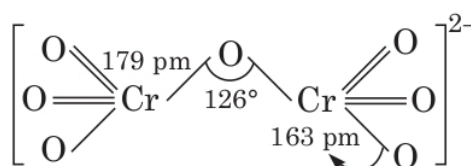
Dichromate ion
